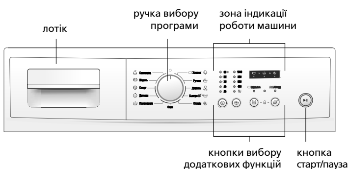
Рисунок 1 – Панель керування
