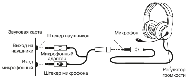
Рис. 1. Схема подключения
