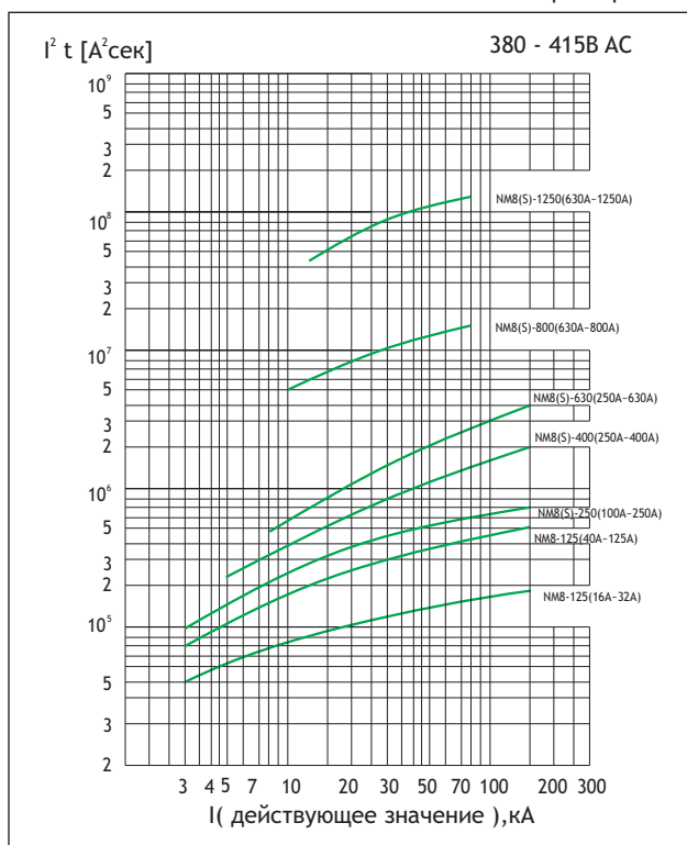
A^2сек характеристика
