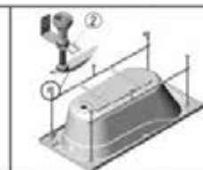
Рисунок 3 - Установка кронштейна для крепления экрана
