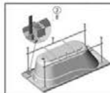
Рисунок 2 - Установка клипсы
