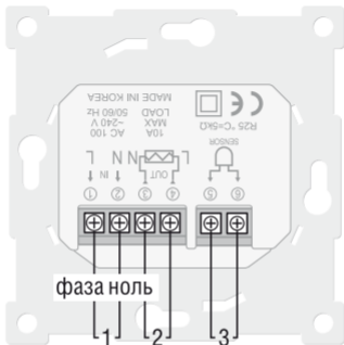
Рис. 2. Схема подключения терморегулятора к сети.
