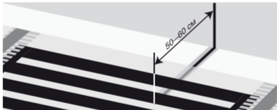
Рис. 1. Схема установки датчика температуры пола
