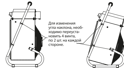
Рис. 2. Тепловентилятор
