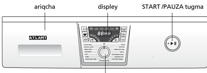
kir yuvish dasturini tanlash dastagi
