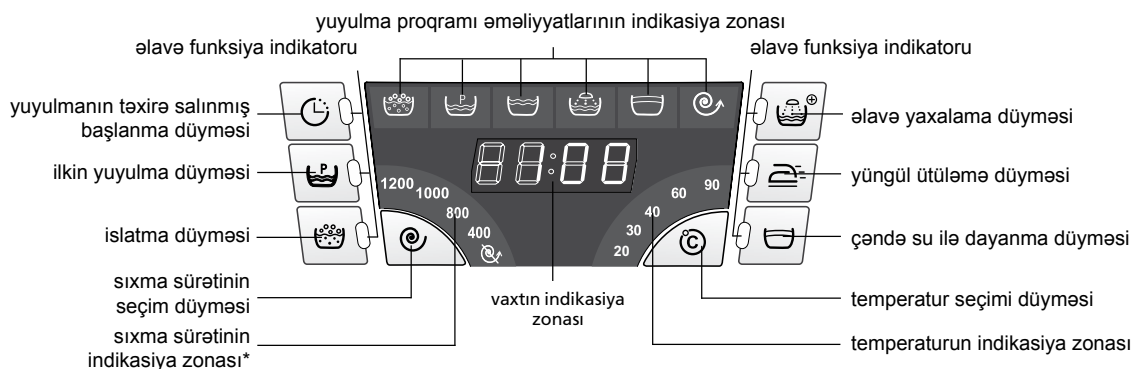
Şəkil 2 – Yuyulma proqramının seçilməsi dəstəyi
