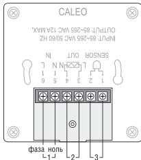
Модели 320/520
