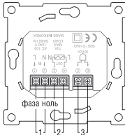
Модель 720
