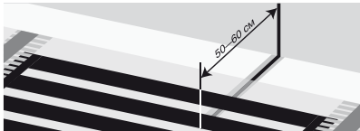
Рис. 5. Схема установки датчика температуры пола
