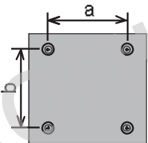
Рисунок 6 – Размеры для выбора настенного кронштейна
