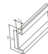
TH35-7.5 DIN rail
