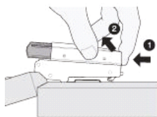
Демонтаж демпфера
