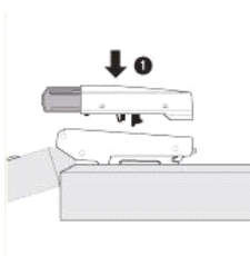
Монтаж демпфера
