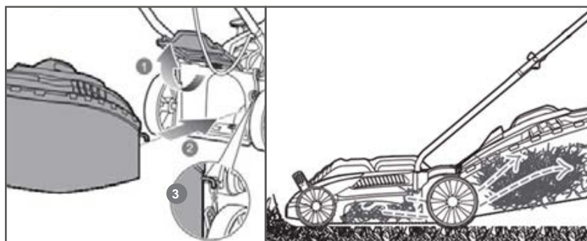
Рис. 6 Установка травосборника
