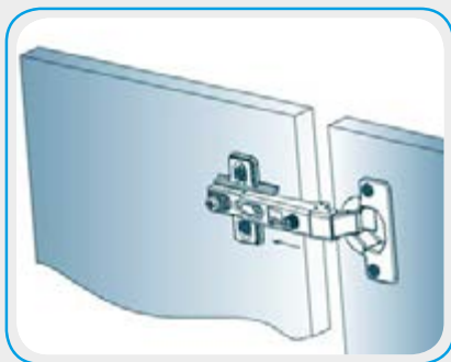
Установка дверной петли
