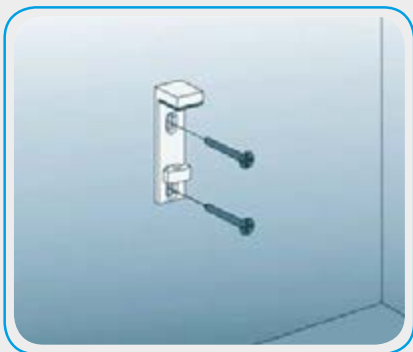
Монтаж планки «Пеликана»
