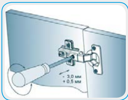
Регулировка наложения навеса
