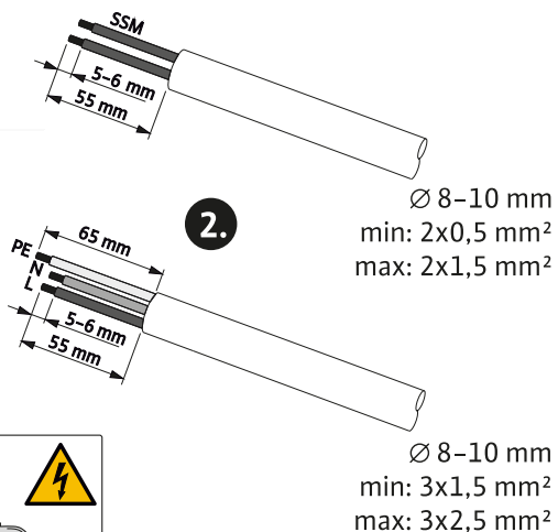
Fig. 15: Подготовка подключения
