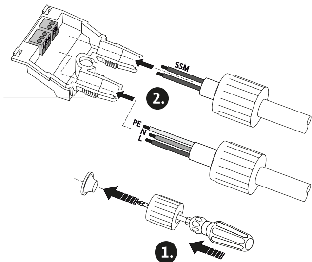
Fig. 18: Электроподключение
