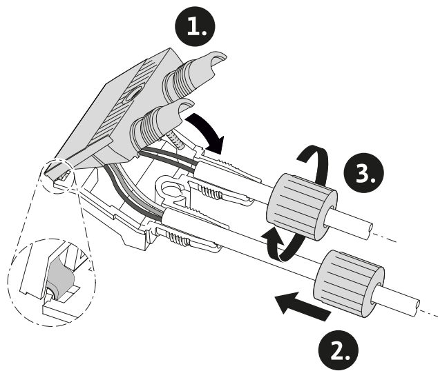
Fig. 20: Закрывание штекера
