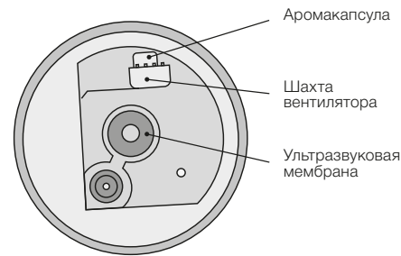
Рис. 3. База прибора
