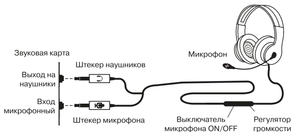
Рис. 1. Схема подключения
