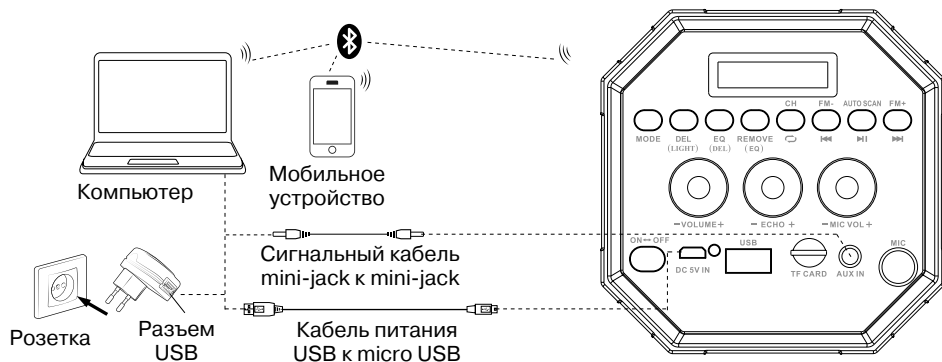
Рис. 2. Схема подключения
