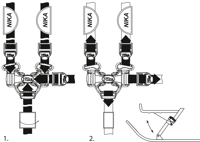
Рис. 3 Крепление ремней безопасности
