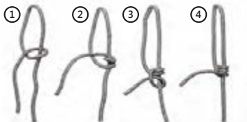
рис. 3 Схема завязывания узла на перемычке санок.
