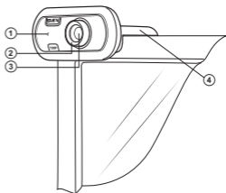
Рис. 1. Устройство веб-камеры
