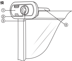
Мал. 1. Будова веб-камери
