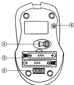
Рис. 2. Вид снизу
