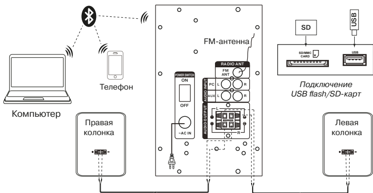
Рис. 5. Схема с подключением Bluetooth-модуля
