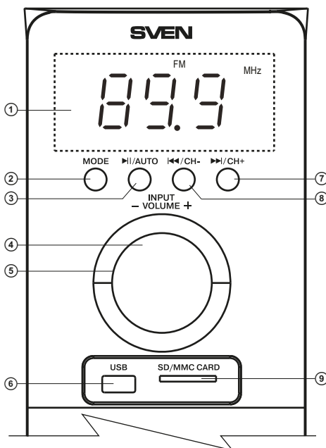
Мал. 1. Панель управління сабвуфера
