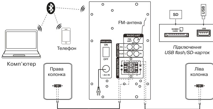
Мал. 5. Схема з підключенням Bluetooth-модуля
