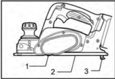
1-нож; 2-задняя часть базы; 3-опора
