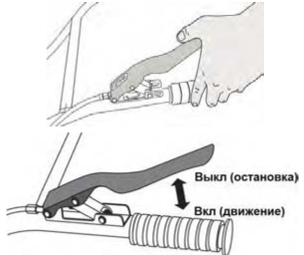
Рисунок 7 – Рычаг сцепления
