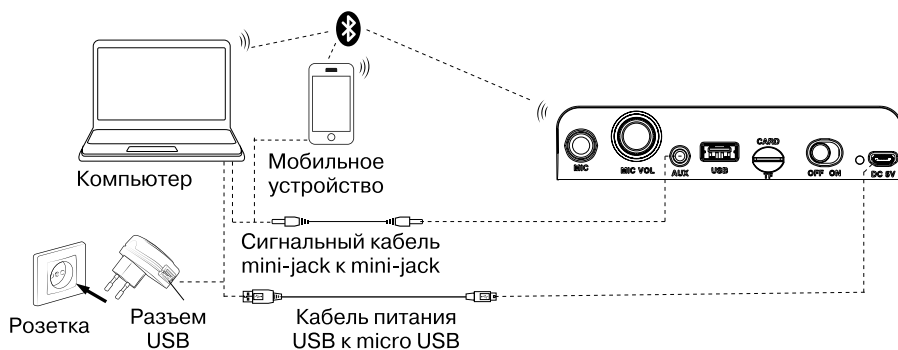
Рис. 3. Схема подключения
