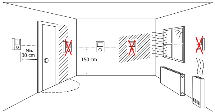
Рисунок 31. Положение термостата
