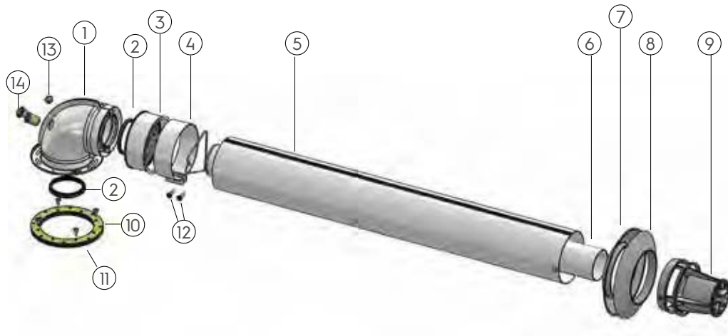
Рисунок 11. Дымоход котла
