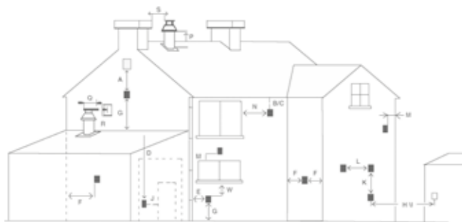
Рисунок 10. Периферийные точки дымохода
