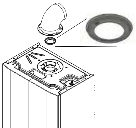
Рисунок 14. Установка редуктора
