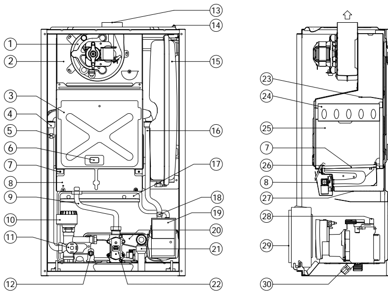
Рисунок 25. Компоненты котла
