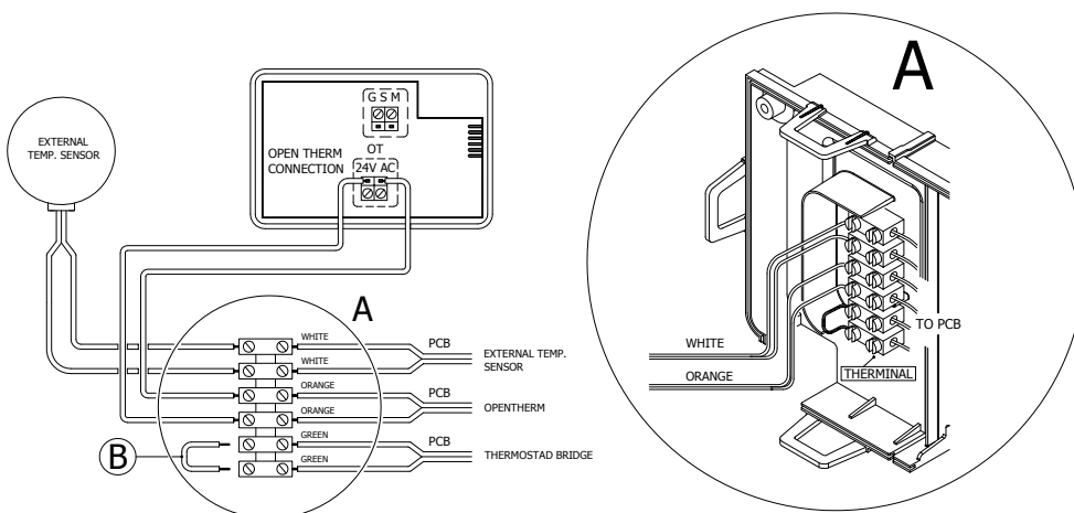
Рисунок 21. Подключение термостата и внешнего датчика погоды
