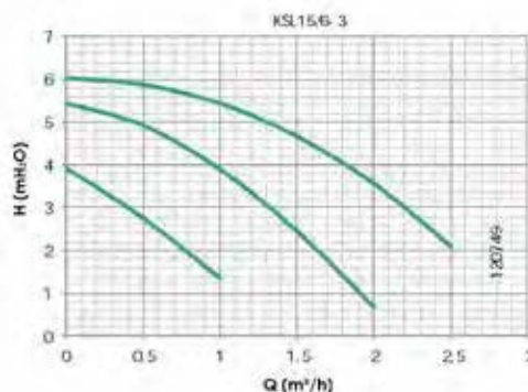
Рисунок 22. Кривая потока / давления насоса
