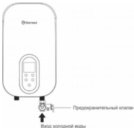
Рис.3 Установка предохранительного клапана
