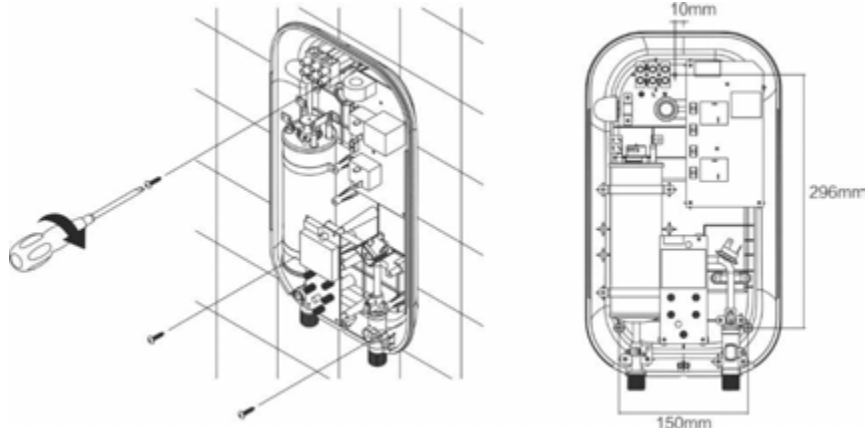
Рис.1 Монтаж ПЭВН на стену
