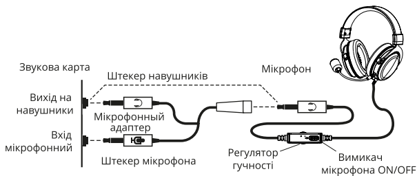
Мал. 2. Схема підключення
