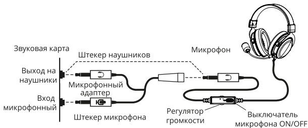
Рис. 2. Схема подключения
