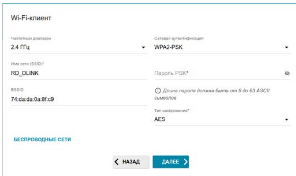
Рисунок 29. Страница настройки Wi-Fi-клиента.
