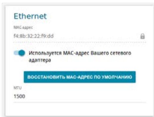
Рисунок 72. Страница добавления соединения типа PPPoE IPv6 . Раздел Ethernet .
