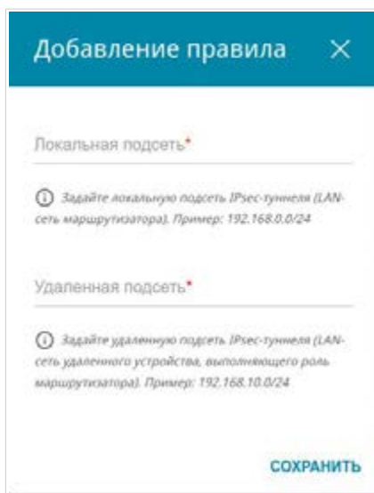
Рисунок 132. Страница добавления IPsec-туннеля. Окно добавления туннелируемой подсети.
