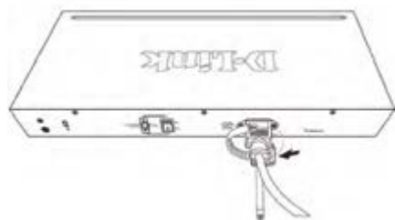
Рисунок 3-4. Фиксация кабеля питания
