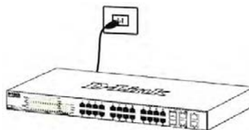
Рисунок 6. Подключение коммутатора к розетке
