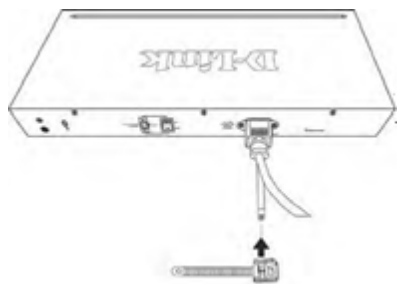
Рисунок 3-3. Установка зажима на стяжку
