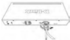
Рисунок 3-4. Фиксация кабеля питания
