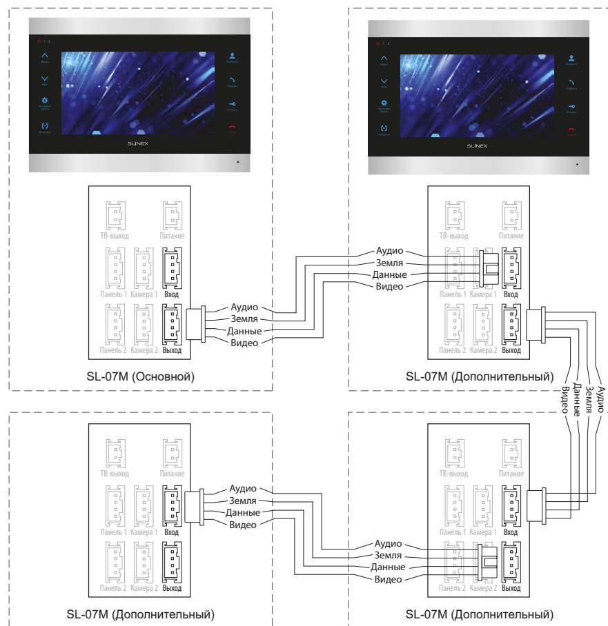
Схема 2. Подключение системы домофонов SL-07M.
