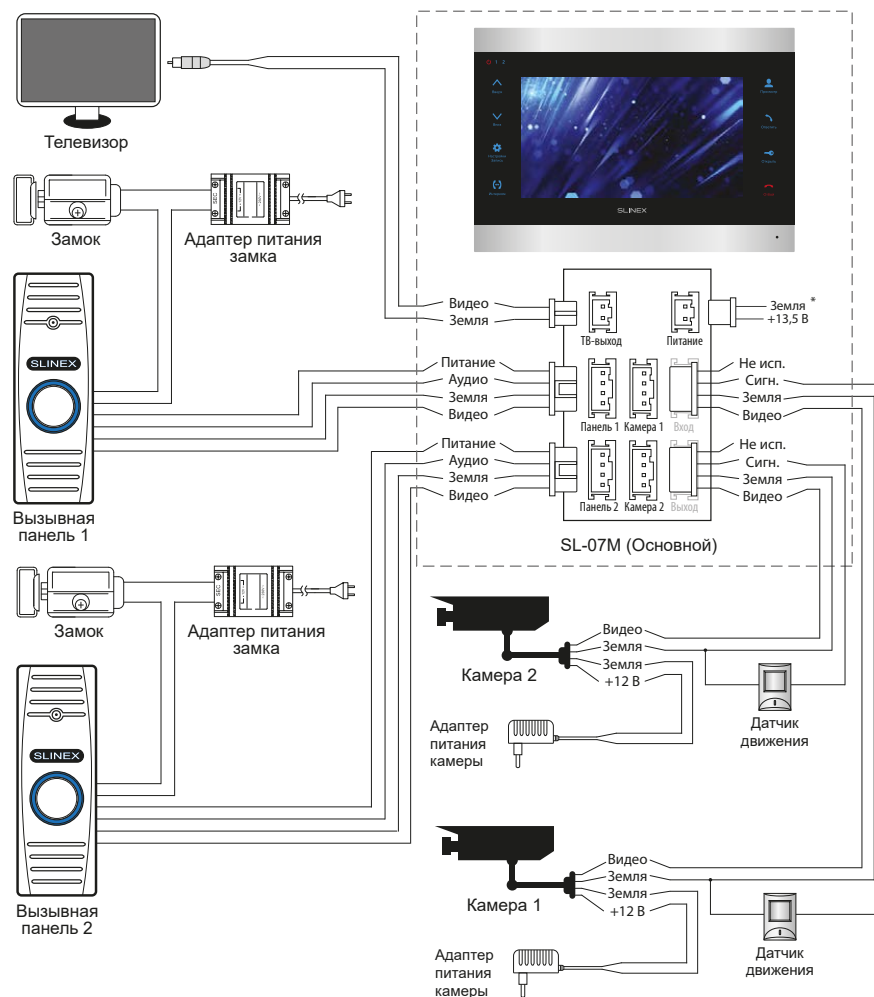
Схема 1. Подключение вызывных панелей, камер и телевизора к домофону SL-07M.
