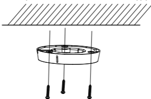
Рисунок 2-12 Установка монтажной платформы
