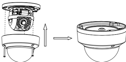
Рисунок 2-9 Установка купола
