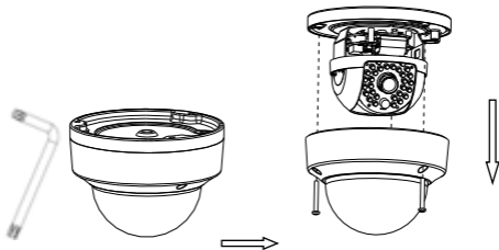
Рисунок 2-5 Демонтаж купола
