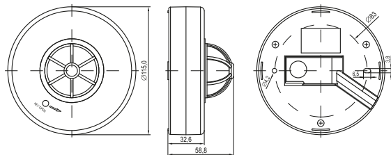
Рисунок 3 – Габаритные размеры
