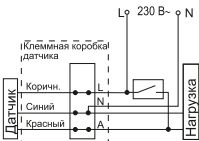
Рисунок 7 – Схема режима с постоянным включением нагрузки
