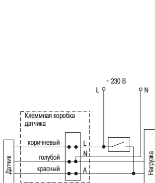
Рисунок 27 – Схема режима постоянного включения нагрузки
