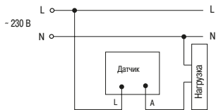
Рисунок 25 – Схема подключения датчика типа ДД 044
