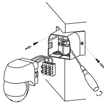
Рисунок 18 – Монтаж ДД 015, ДД 016
