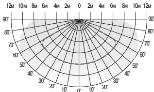
Рисунок 1 – ДД 013, ДД 015, ДД 016
