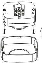
Рисунок 19 – Монтаж ДД 022, ДД 023
