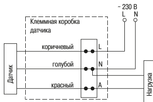
Рисунок 24 – Схема подключения датчиков типов ДД 022, ДД 023
