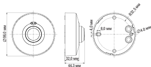
Рис. 2. Габаритные и установочные размеры MW-703
