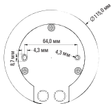
Рис. 3. Габаритные и установочные размеры MW-705
