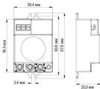
Рис. 4. Габаритные и установочные размеры MW-706
