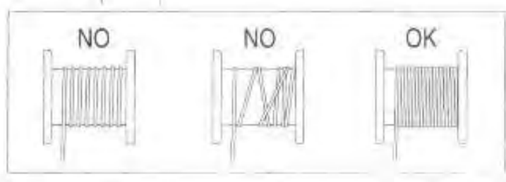
Рис.6 - Намотка троса на катушку
