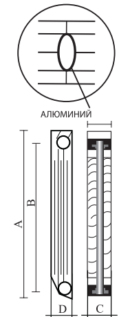
Чертежи радиатора в разрезе
