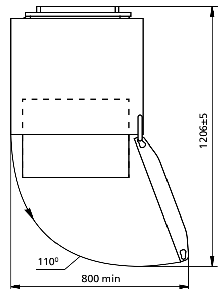
Рисунок 2 – Холодильник (вигляд зверху)
