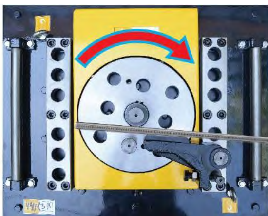
Подача справа
