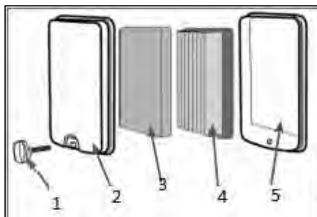
Рис. 20 Обслуживание воздушного фильтра Т-50
