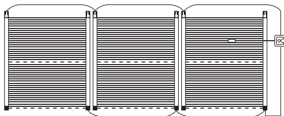
Рисунок 1. Общая схема подключения, в случаях, когда установочные провода проложены под плинтусом, утоплены в прорезях теплоизоляции, или в специальных кабель-каналах, исключающих непосредственное механическое воздействие.
