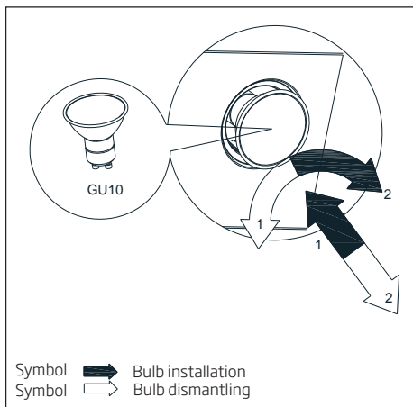
Obr. 11 Výmena osvetlenia
