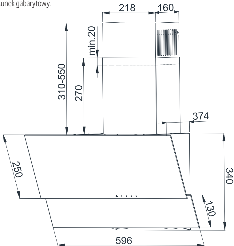
Rys.2 Rysunek gabarytowy.
