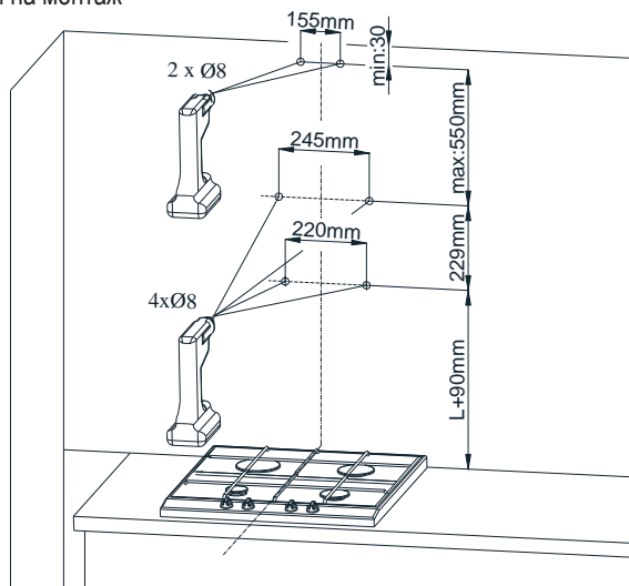
Фиг. 4 Размери на монтаж
