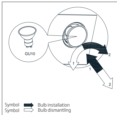
Fig.11 Înlocuirea iluminatului
