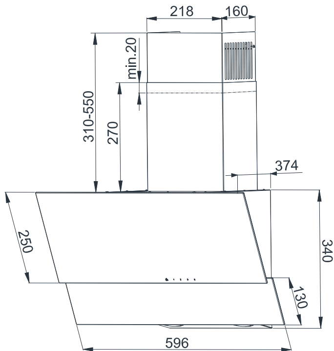
Obr.2 Kresba rozměrů
