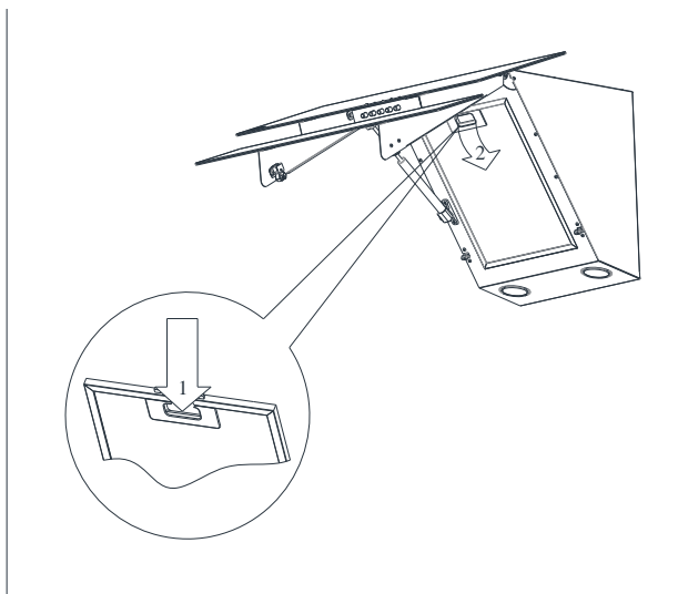
Rys. 7 Demontaż filtra aluminiowego przeciwzapalnego.
