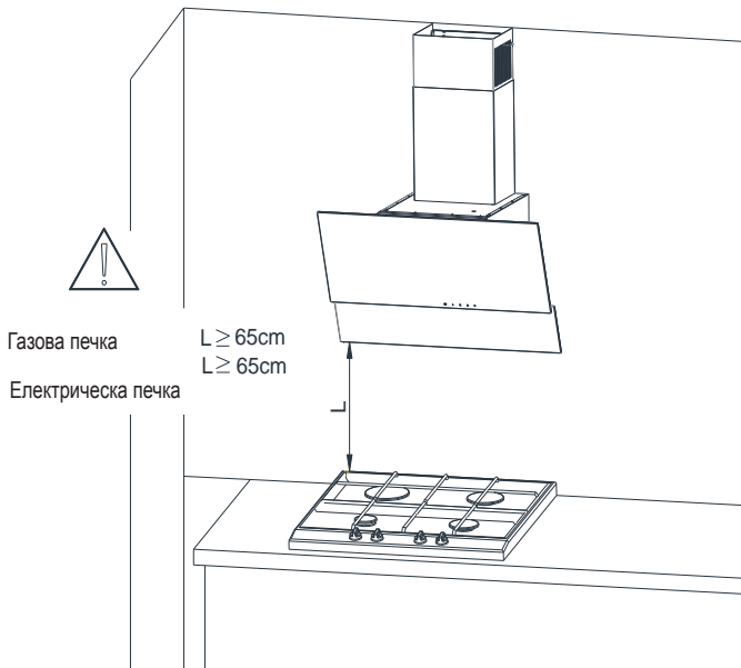
Фиг. 3 Примерно разстояние от кухненска та печка
