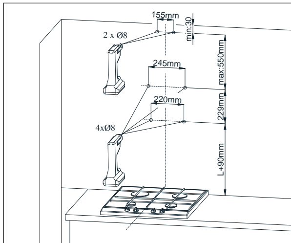
Rys. 5 Montaż kołków rozporowych.
