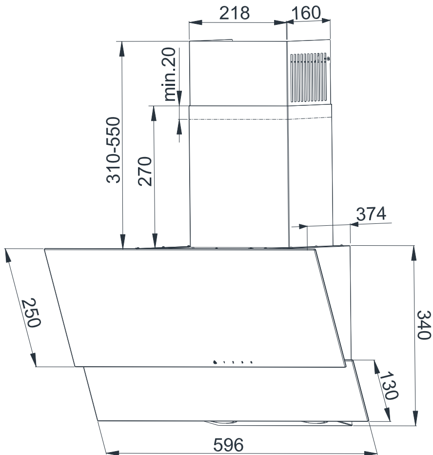
Abb. 2 Dimensionszeichnung
