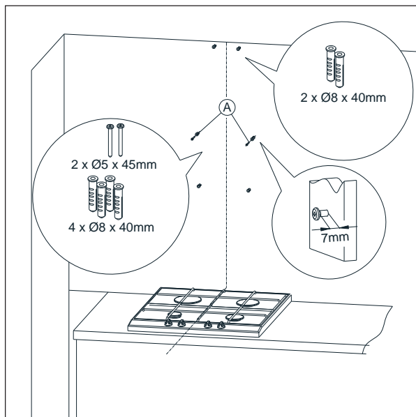
Abb. 5 Spreizschrauben montieren
