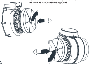
Фиг. 10 Смяна на въглеродния филтър
