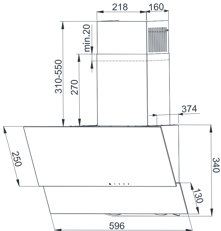
Obr.2 Rozmer kreslenia
