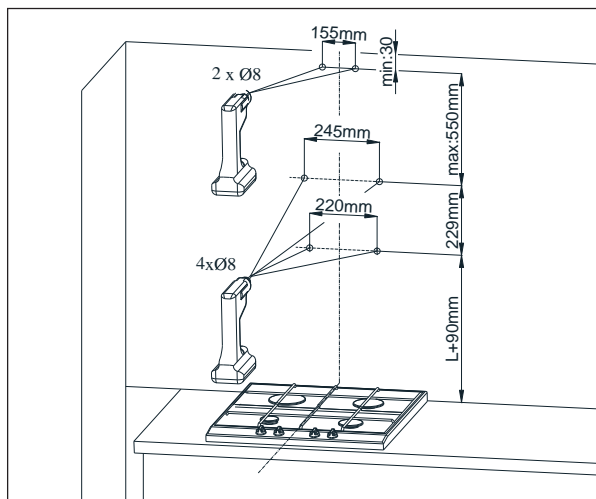
Abb. 5 Spreizschrauben montieren
