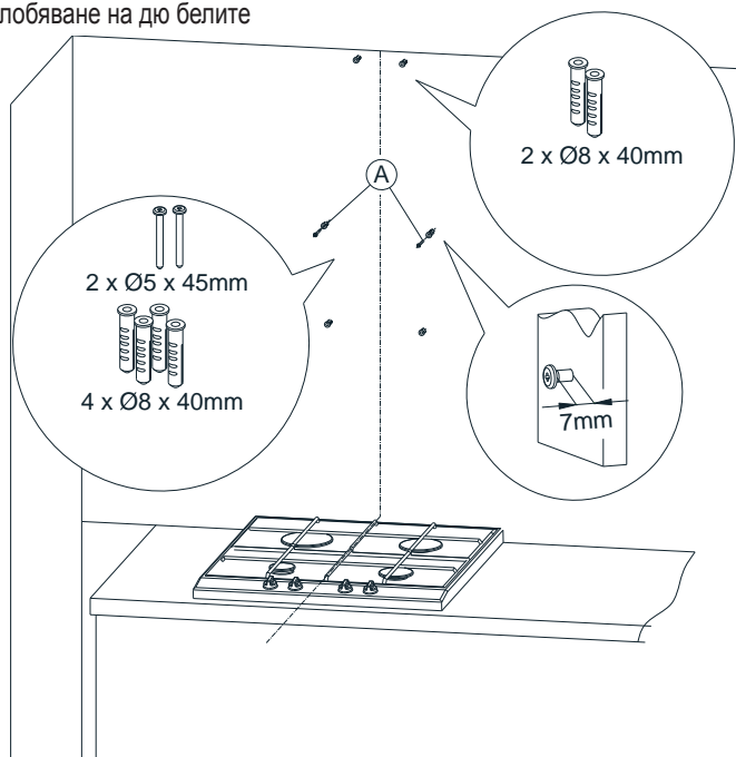
Фиг. 5 Сглобяване на дюбелите
