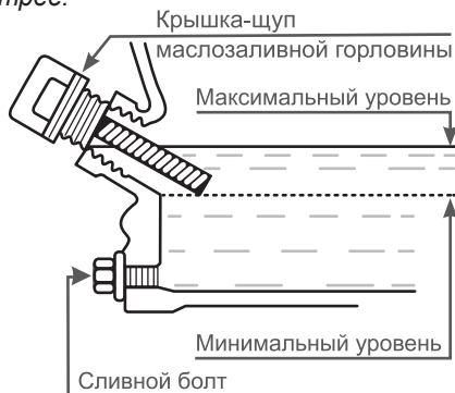
Рис. 20 Замена моторного масла
