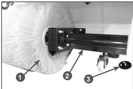
Рис. 25 Снятие щетки
