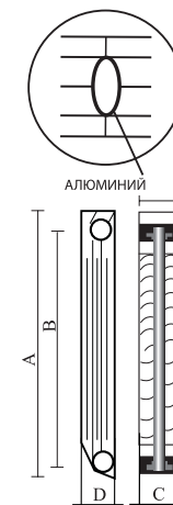
Чертежи радиатора в разрезе
