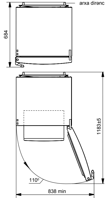
Şəkil 2 – Dondurucu (yuxarıdan görüntü)
