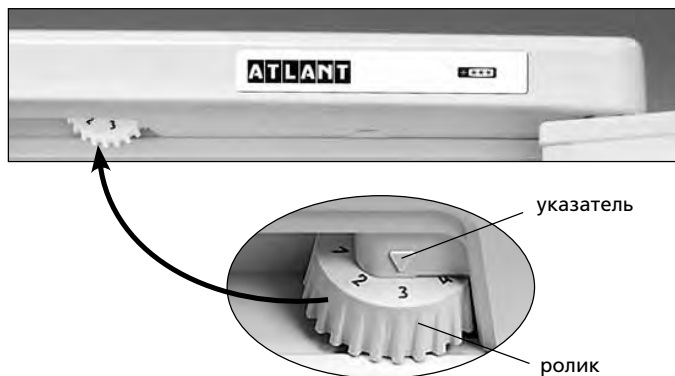
Рисунок 3 – Регулировка температуры
