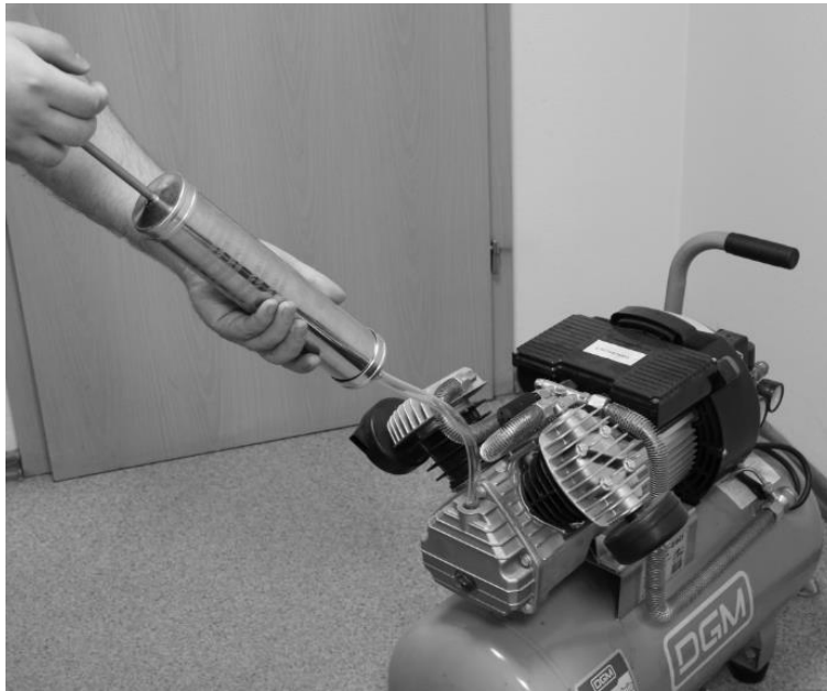
Рисунок 3 – Замена масла
