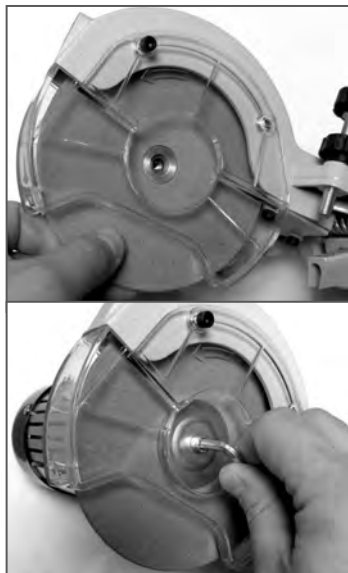
Рис. 5 Установка заточного диска
