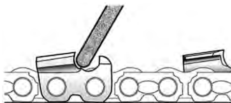
Рис. 16 Регулировка глубины заточки
