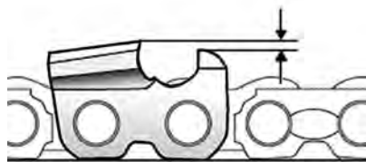
Рис. 22 Глубина резания
